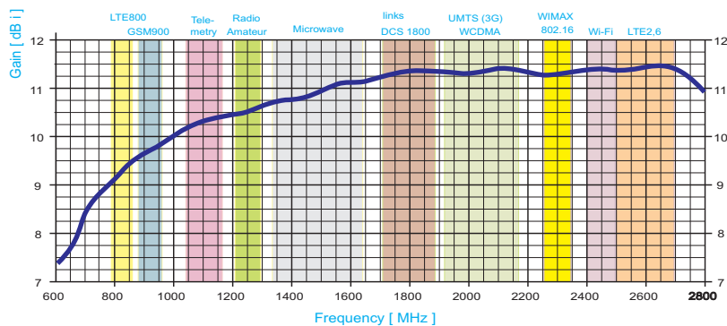
Antenne LAT-56
